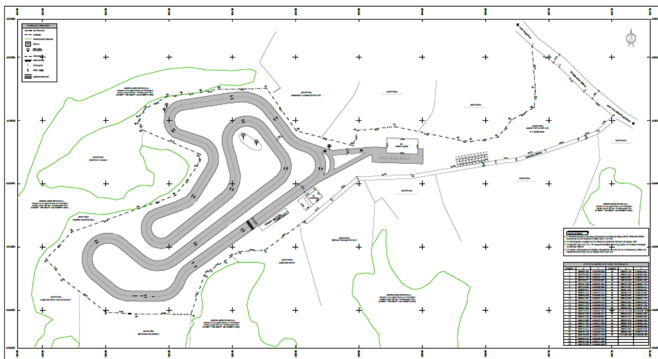
Χάρτης 1 : Τοπογραφική αποτύπωση Πίστας Καρτ
