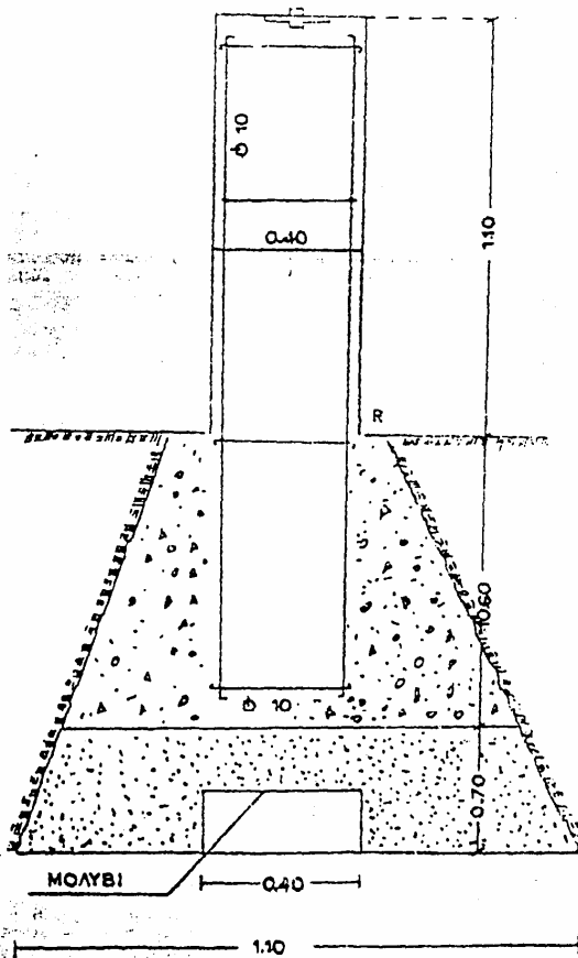
ΣΧΗΜΑ 1 ΣΗΜΑΝΣΗ ΣΗΜΕΙΟΥ ΟΡΙΖΟΝΤΙΟΓΡΑΦΙΚΟΥ ΕΛΕΓΧΟΥ Εκ σκυροκονιάματος πλάξ άρειχαλκίνη
