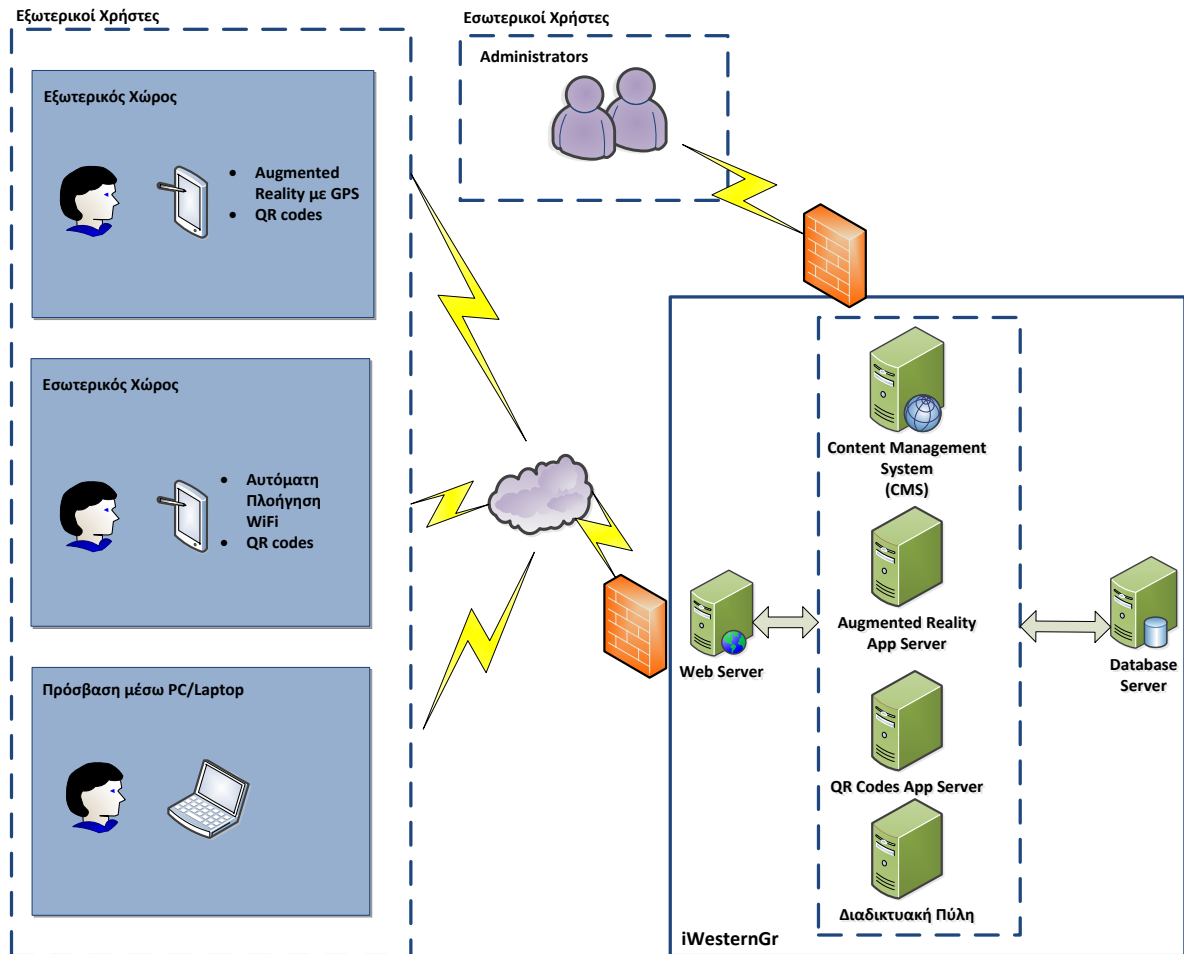
Σχήμα 1 : Λογική Αρχιτεκτονική
