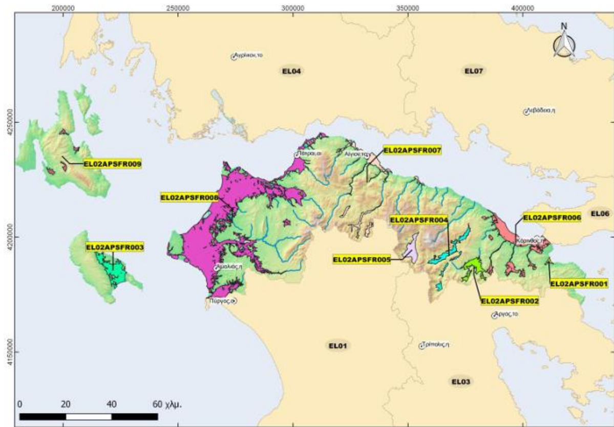
Εικόνα 5: Απόσπασμα του Χάρτη αποτίμησης των Ζωνών Δυνητικά Υψηλού Κινδύνου Πλημμύρας- Υδατικό Διαμέρισμα Βόρειας Πελοποννήσου (EL02) βάσει της 1ης Αναθεώρησης της ΠΑΚΠ.
